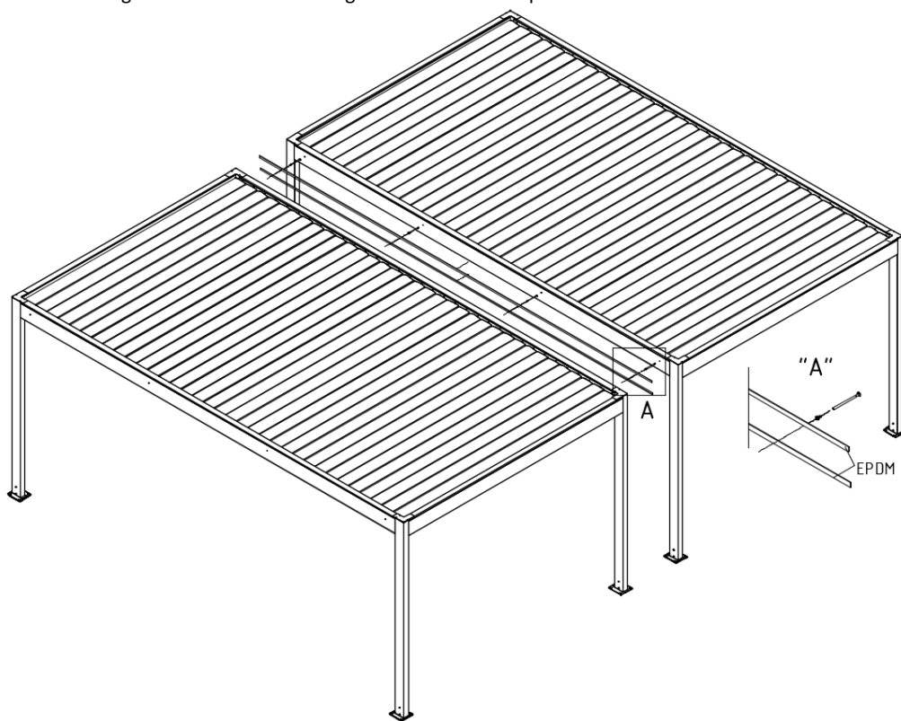
Fig. 4b. Vue de l'assemblage des modules de la Pergola SB400PRO
