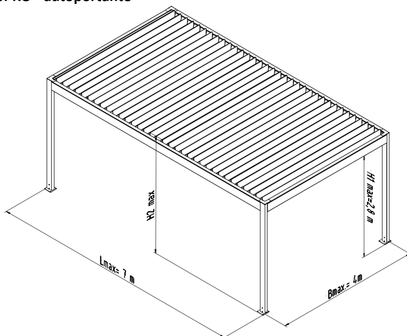
Fig. 1. Pergola SB400PRO autoportante - Dimensions hors tout: B max – largeur maximale, L max – longueur maximale, H max – hauteur maximale du cadre (3048 mm), H1 max – passage libre du cadre, H2 max – hauteur maximale de position du mécanisme de changement de l'angle des lames (~3095 mm).
