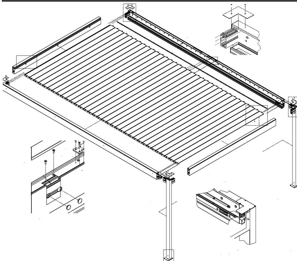
Fig. 5a. Vue de l'assemblage de la Pergola SB400PRO- murale (transversale).
