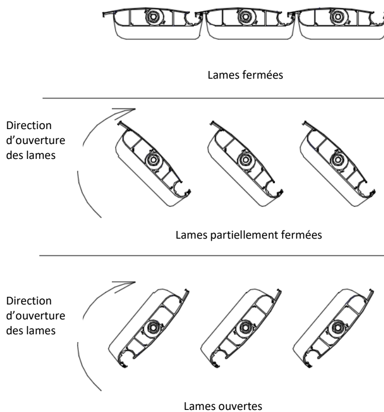
Fig. 3 Réglage standard du sens d'ouverture des lames pour la Pergola SB400PRO
