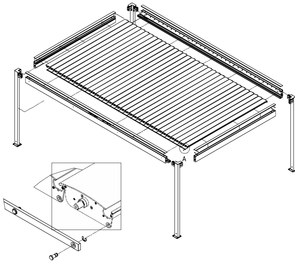
Fig. 4a Vue de l'assemblage des éléments de la Pergola SB 400PRO autoportante
