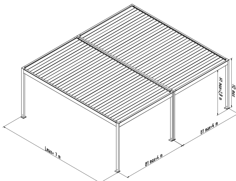
Fig. 2. Pergola SB400PRO modulaire – Dimensions hors tout: B max – largeur maximale, L max – longueur maximale, H max – hauteur maximale du cadre (3048 mm), H1 max – passage libre du cadre, H2 max – hauteur maximale de position du mécanisme de changement de l'angle des lames (~3095 mm).
