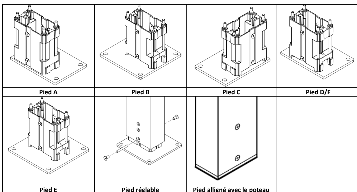
Fig. 7. Types des pieds Pergola SB400PRO.
