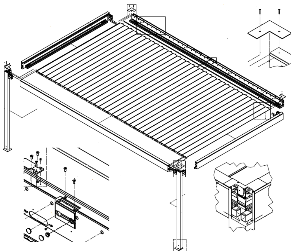
Fig. 5b.). Vue de l'assemblage de la Pergola SB400PRO- murale (perpendiculaire).
